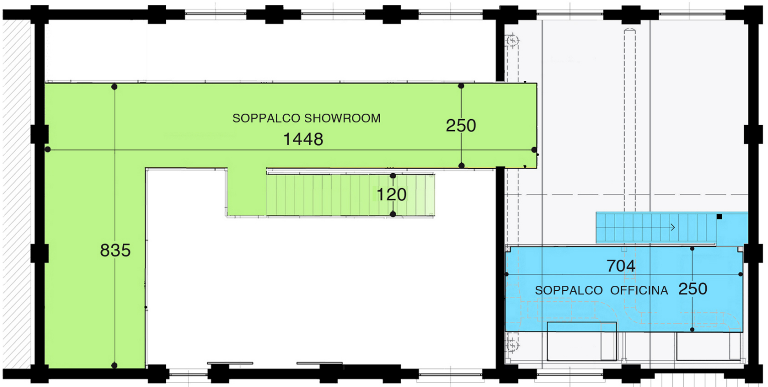
PIANTA SOPPALCO
